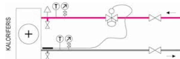
Oro užuolaidos mazgas
