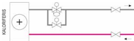
Oro užuolaidos mazgas vartams
