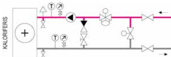
Oro vėdinimo kameros aprišimo mazgas šildymui
