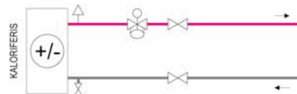
Ventiliatorinio konvektoriaus arba oro šildytuvo aprišimo schema vėsinimui arba šildymui
