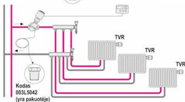
Grindinio šildymo sistema su pagrindiniu reguliatoriumi
