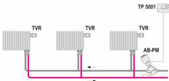
Radiatorių šildymo sistema, naudojant elektroninį kambario termostatą
