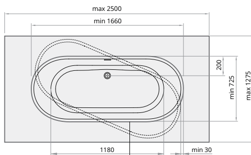
minimalus paviršius
